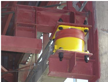
Соединение демпферами ВД двух соседних зданий, имеющих различную массу, собственные частоты и формы вынужденных колебаний
